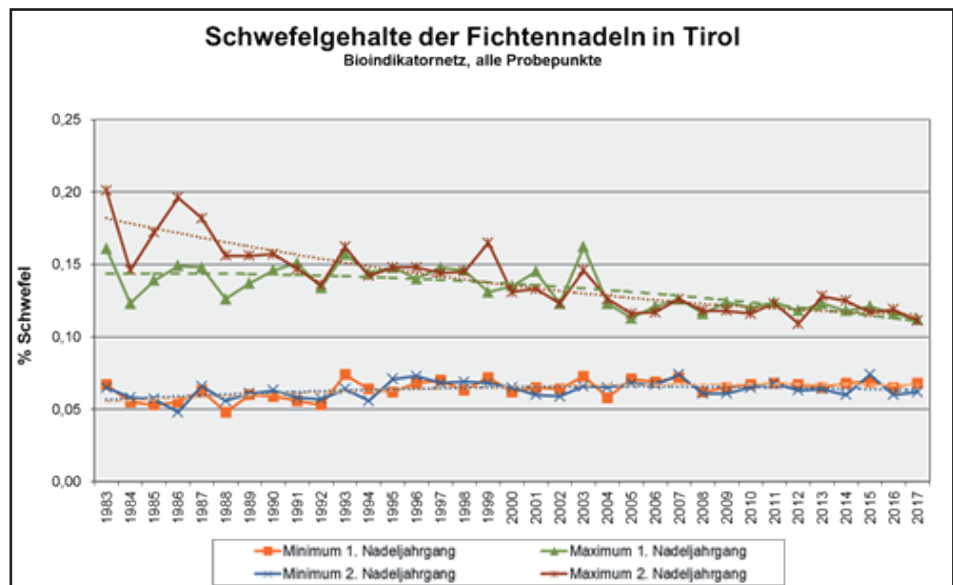
Abb. II.4.3.1: Minimale und maximale Schwefelgehalte von Fichtennadeln im Bioindikatornetz, 1983 bis 2017. (Gruppe Forst)
