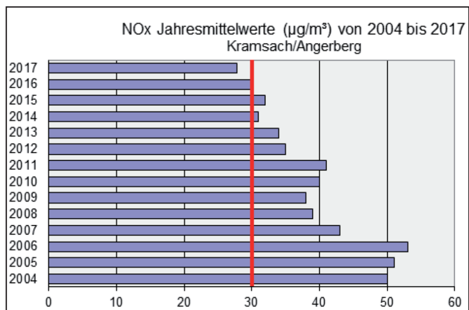
Abb. II.4.1.1: Entwicklung der Stickoxidbelastung an der Messstelle Kramsach/Angerberg, 2004 bis 2017. Die rote Linie markiert den Jahresmittelgrenzwert von 30 µg/m 3 nach IG-L. (Gruppe Forst)
