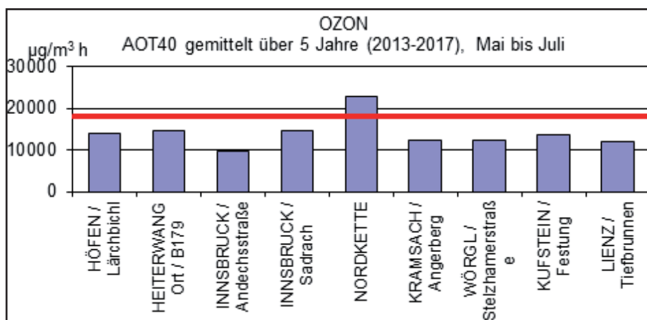
Abb. II.4.1.2: Ozonbelastung 2017 ausgedrückt als AOT40-Wert zum Schutz der Vegetation an den Messstellen des Tiroler Luftgütemessnetzes. (Gruppe Forst)
