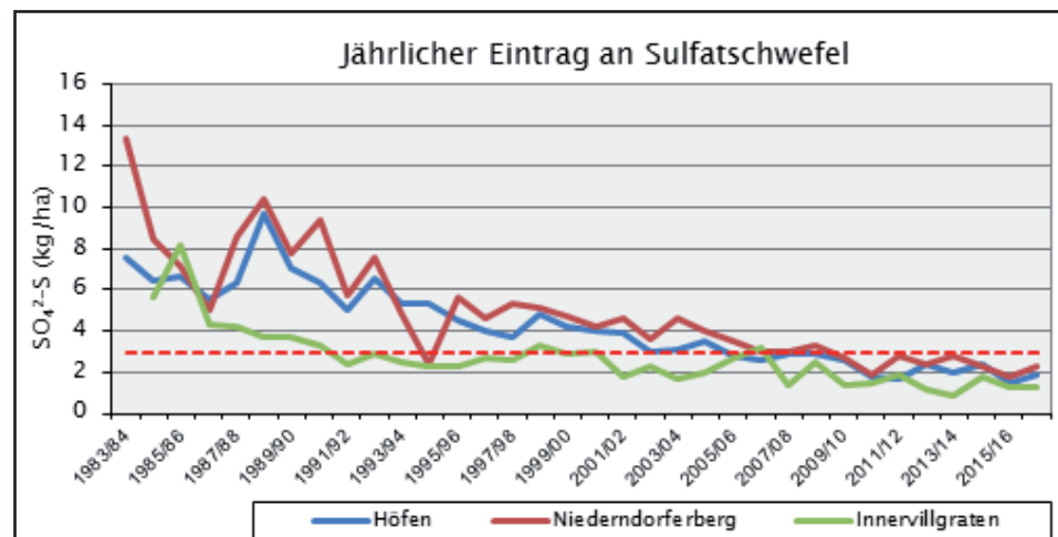
Abb. II.4.2.1: Jährlicher Eintrag an Sulfatschwefel an den Messstellen Höfen/Reutte, Niederndorferberg/ Kufstein und Innervillgraten/Lienz seit Beginn der Messungen, 1983/84 bis 2016/17. Die rote strichlierte Linie markiert den Grenzwert nach dem „Critical Loads Konzept“. (Gruppe Forst)
