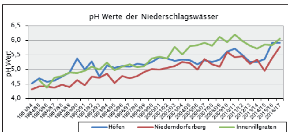
Abb. II.4.2.3: Entwicklung der pH-Werte in den Niederschlagswässern (Regen und Schnee) an den drei Tiroler Messstellen seit Beginn der Messungen, 1983/84 bis 2016/17. (Gruppe Forst)
