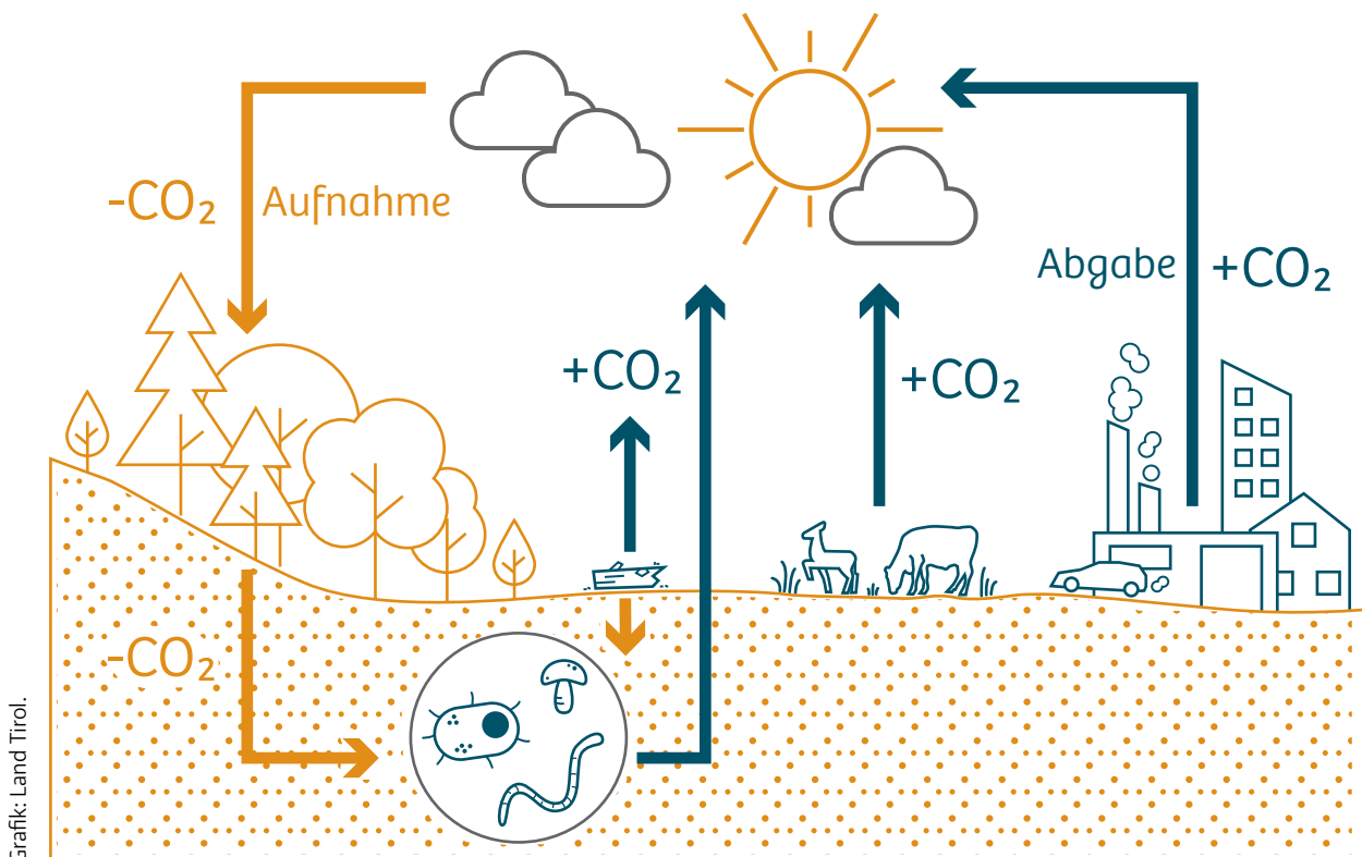
Abb. 4.1: Der Kohlenstoffkreislauf in vereinfachter Darstellung:
